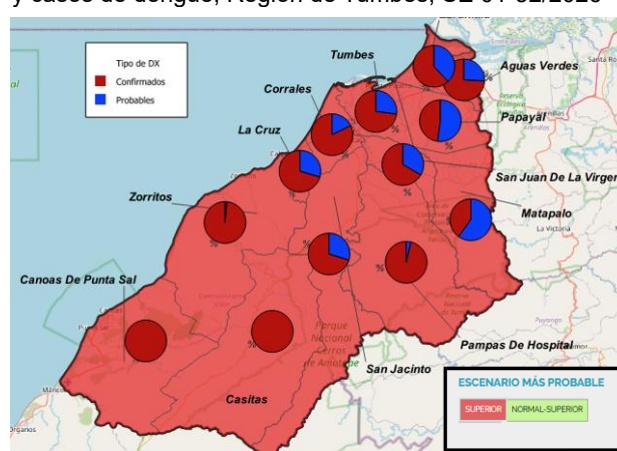
Gráfico 3. Pronóstico climático de temperatura máxima y casos de dengue, Región de Tumbes, SE 01-32/2026
